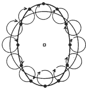
Generación de una órbita elíptica mediante movimientos circulares.
