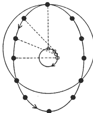
Órbita generada excéntricamente, equivalente desde un punto de vista geométrico.
