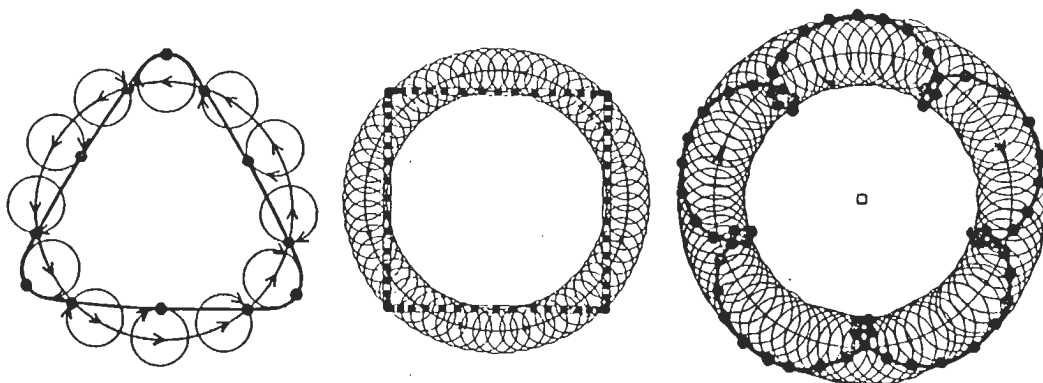
'Orbita' cuadrada a partir de la epiciclicidad.
