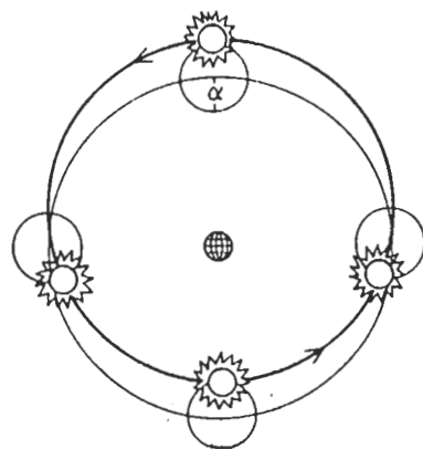
Explicación epicíclica de Hiparco de las estaciones.
