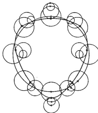
'Órbita oviforme' de Kepler a partir de epiciclos.
